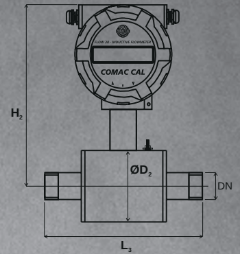
THREAD (EN 10226-1)
